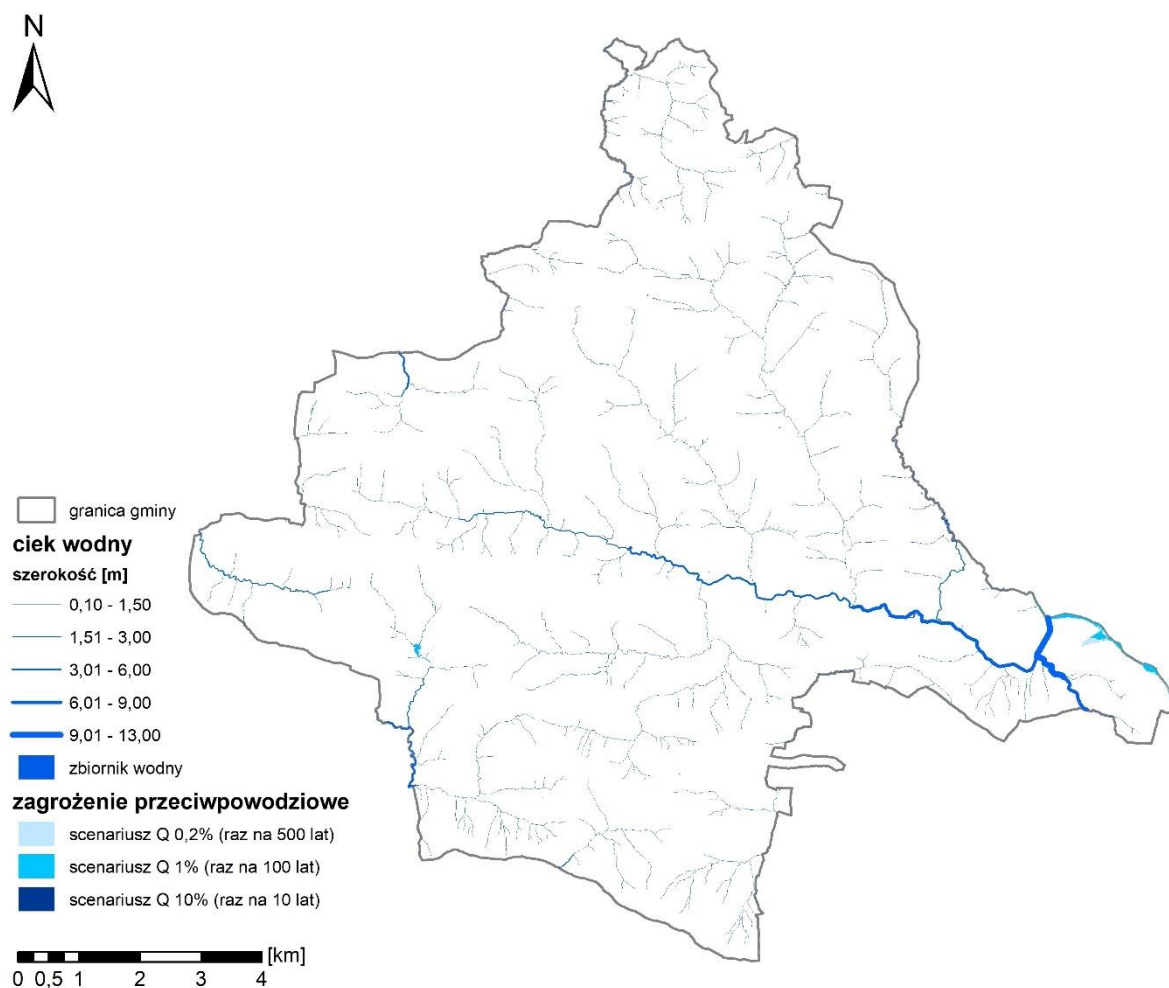
Mapa 4 Obszary szczególnego zagrożenia powodziowego
